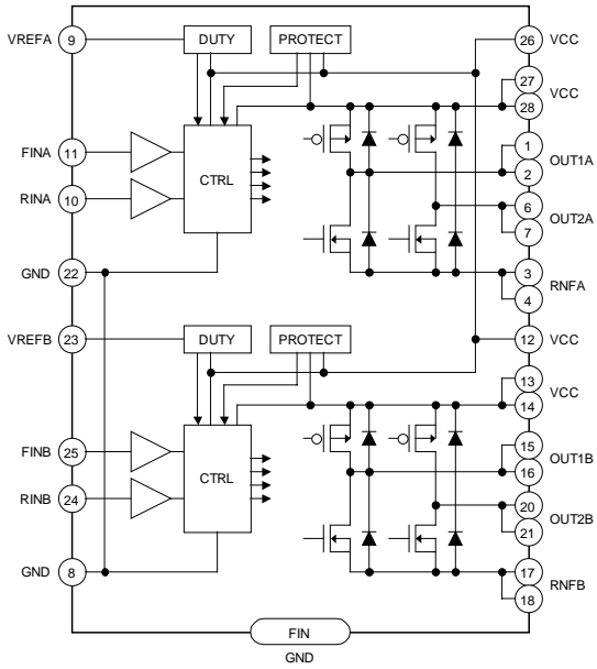
Fig. 36 BD6237FM
